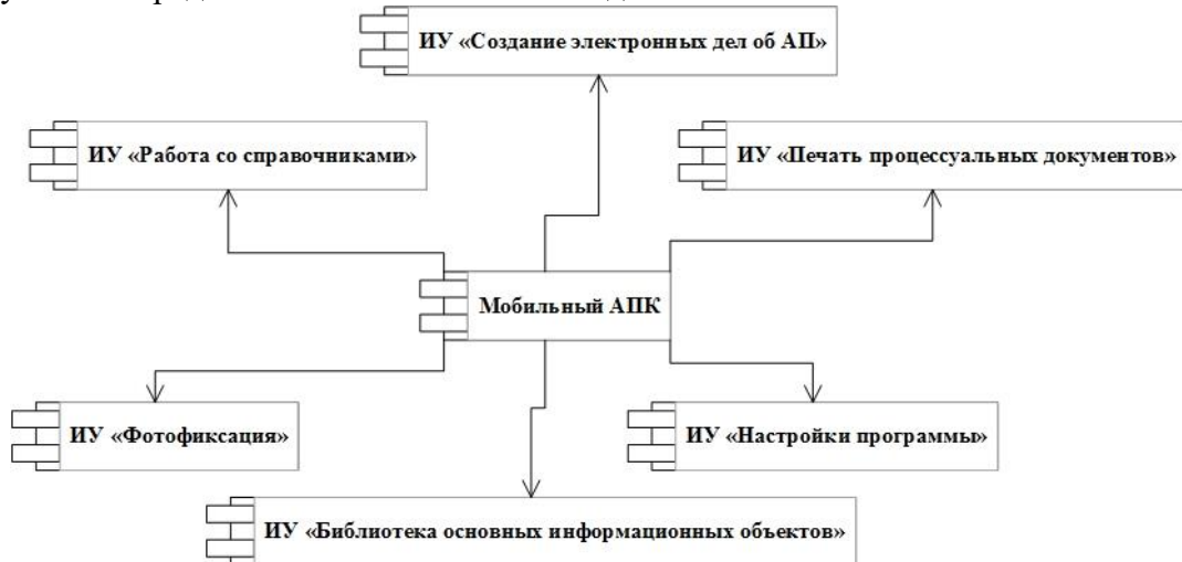
Рисунок 3-2. Компонентная модель Мобильного АПК
